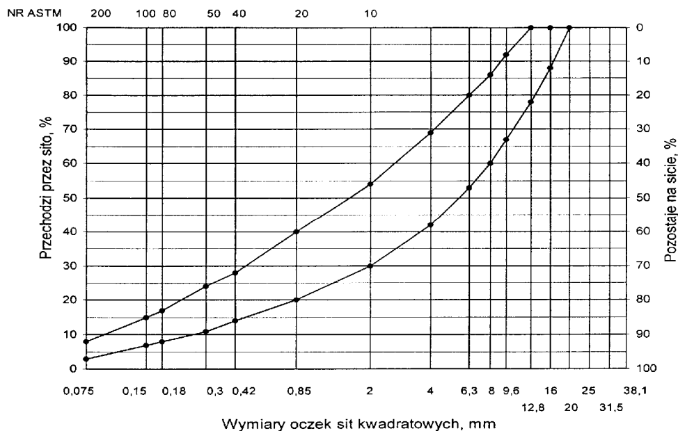
Rys. 8. Krzywe graniczne uziarnienia mieszanki mineralnej BA od 0 do 16mm do warstwy wyrównawczo wzmacniającej
