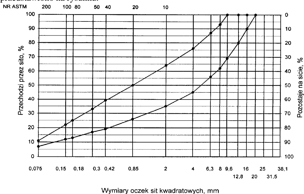
Rys. 3. Krzywe graniczne uziarnienia mieszanki mineralnej BA od 0 do 12,8mm,
