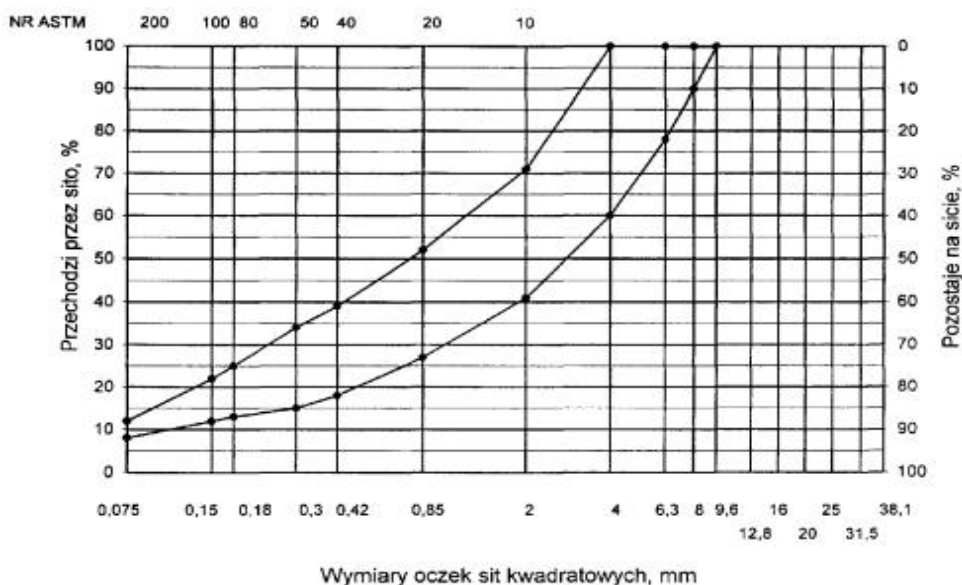
Rys. 3. Krzywe graniczne uziarnienia mieszanki mineralnej BA od 0 do 8mm,
